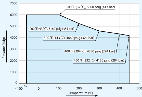
VUH-941 Serie PTFE Packing Type
