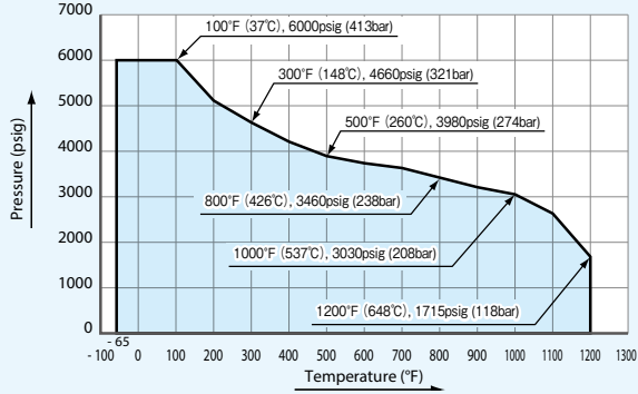
VUH-941 Serie Grafoil Packing Type
